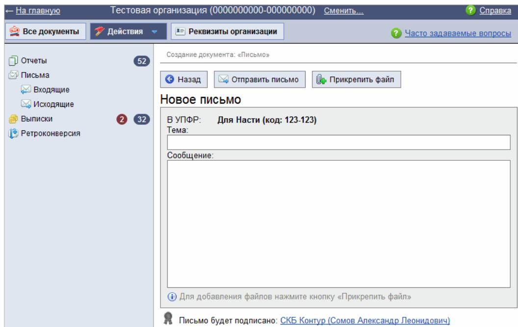
Рис. 10. Создание письма
