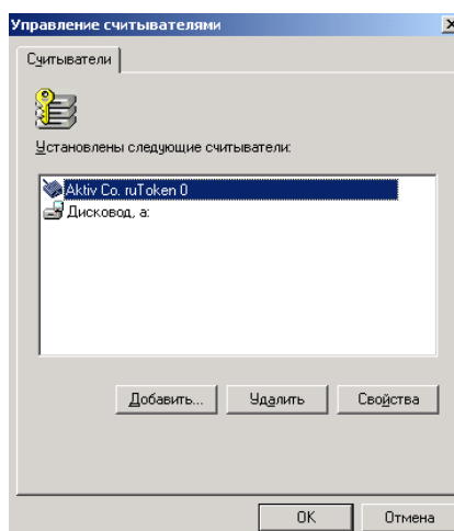
Рис. 28. Управление считывателями
