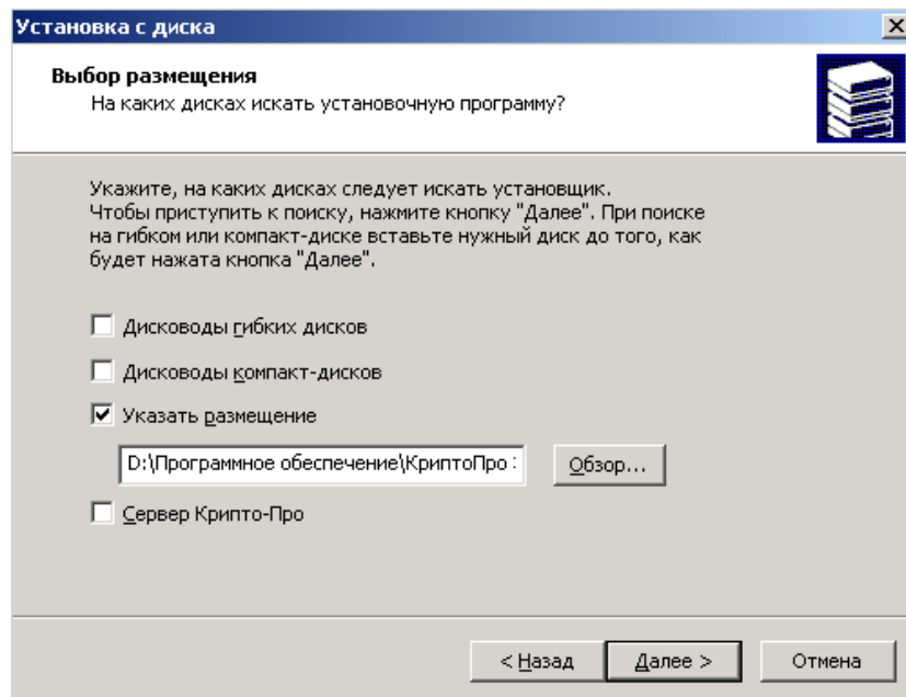
Рис. 23. Выбор размещения
