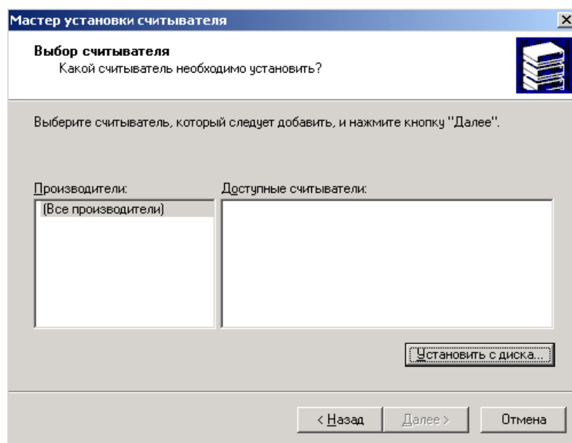
Рис. 22. Выбор считывателя
