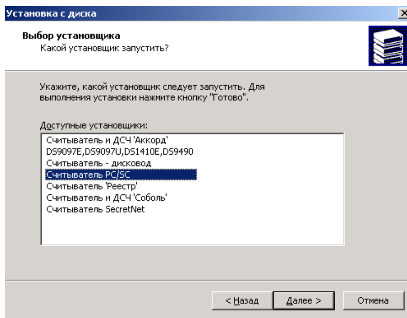
Рис. 24. Выбор установщика
