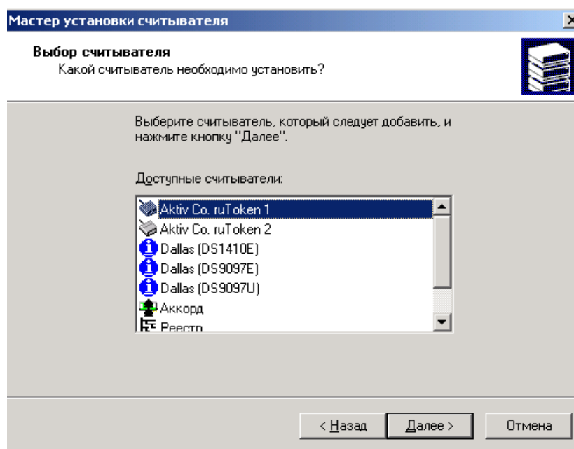
Рис. 29. Выбор считывателя
