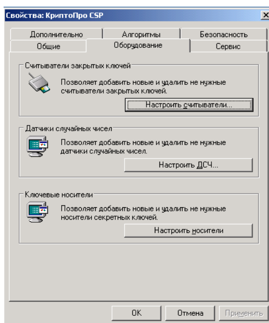
Рис. 20. Вкладка «Оборудование»
