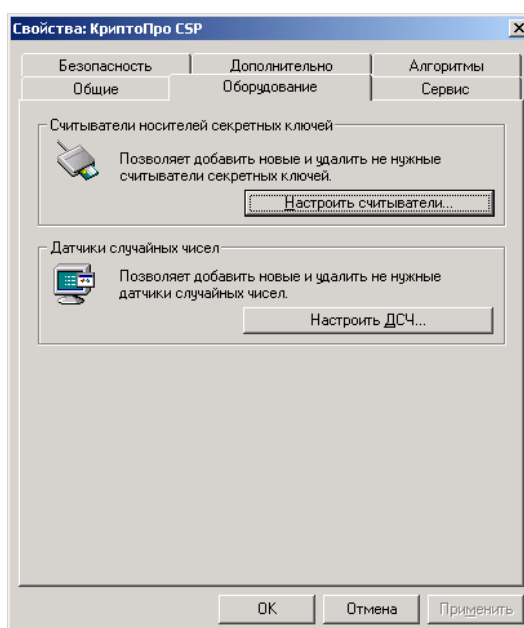
Рис. 27. Вкладка «Оборудование»
