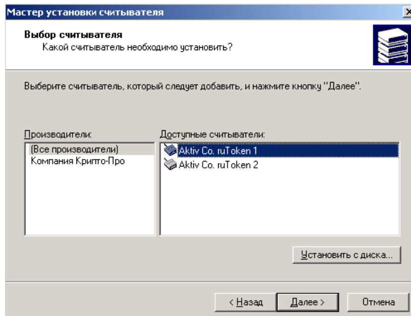
Рис. 25. Выбор считывателя
